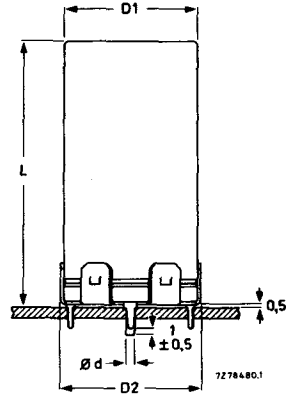
Fig. 2 Style 2; see Table 1b for dimensions d, D1, D2, D3 and L.
