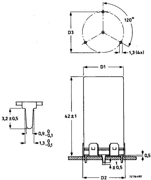
Fig. 2 Style 2; see Table 1b for dimensions D1, D2, D3.
